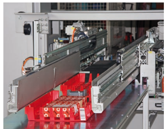
Bild 2: Das Lastaufnahmemittel Viper ist für das Handling von Behältern und Kartons konzipiert
